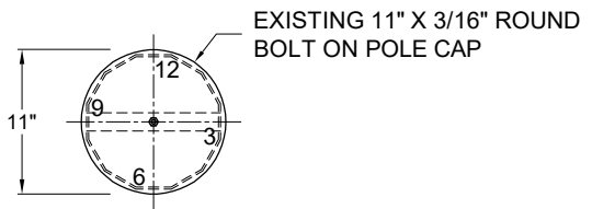
SECTION A-A POLE CAP
