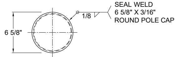
SECTION A-A POLE CAP
