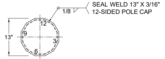
SECTION A-A POLE CAP
