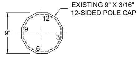
SECTION A-A POLE CAP
