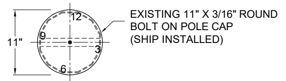
SECTION A-A POLE CAP
