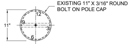
SECTION A-A POLE CAP
