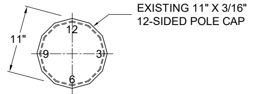
SECTION A-A POLE CAP
