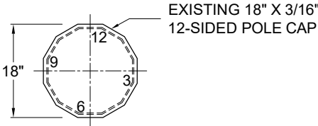
SECTION A-A POLE CAP
